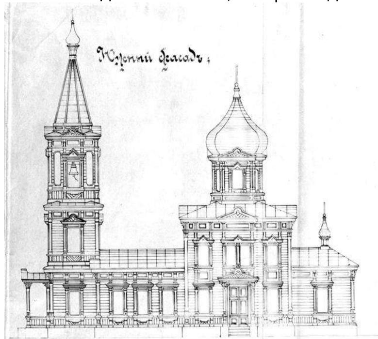
Чертежи православного храма с.Пензенка, 1904 г. (Источник: Центральный государственный архив Самарской области)
